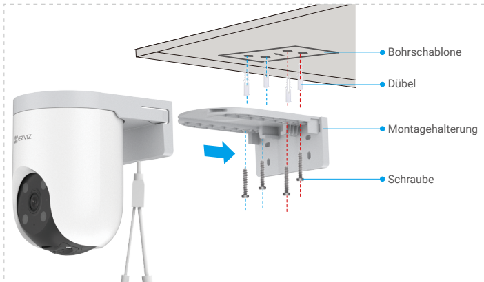
Abb. 1 Deckenmontage
